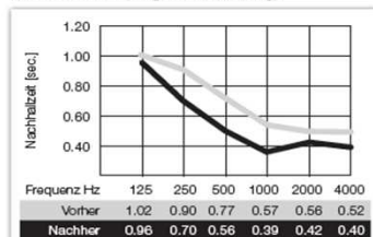
Nachhallzeit (Gegenüberstellung)
